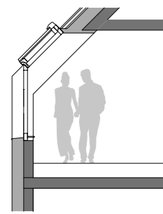
SCHNITT A
